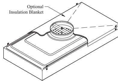
Optional Thermal Insulation
